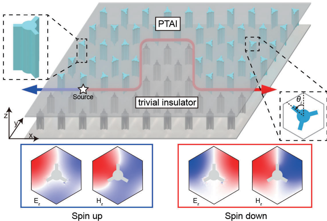
<시간 역전 대칭 광학 토폴로지 앤더슨 절연체의 개략도(청색 부분)>
